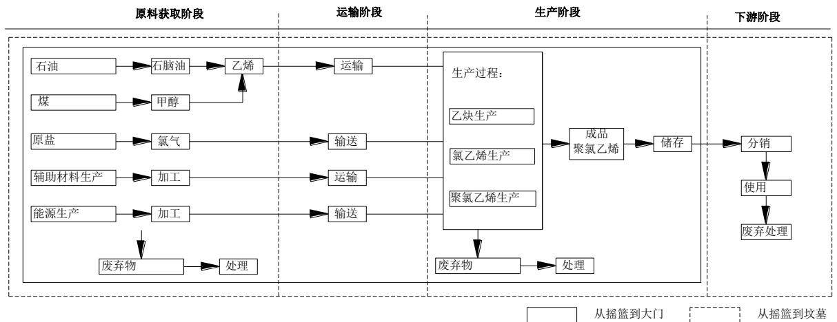
图1-2 乙烯法聚氯乙烯产品生命周期系统边界
