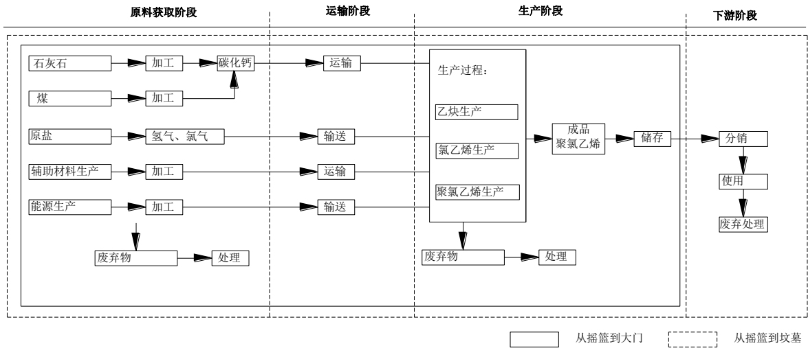
图1-1 电石法聚氯乙烯产品生命周期系统边界
